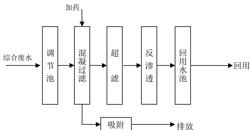
图4 钛白粉生产企业废水深度处理工艺流程图
