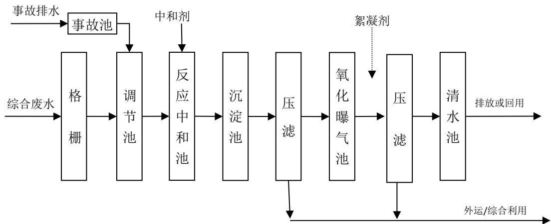
图2 硫酸法钛白粉生产企业废水一级中和二次压滤法处理工艺流程图
